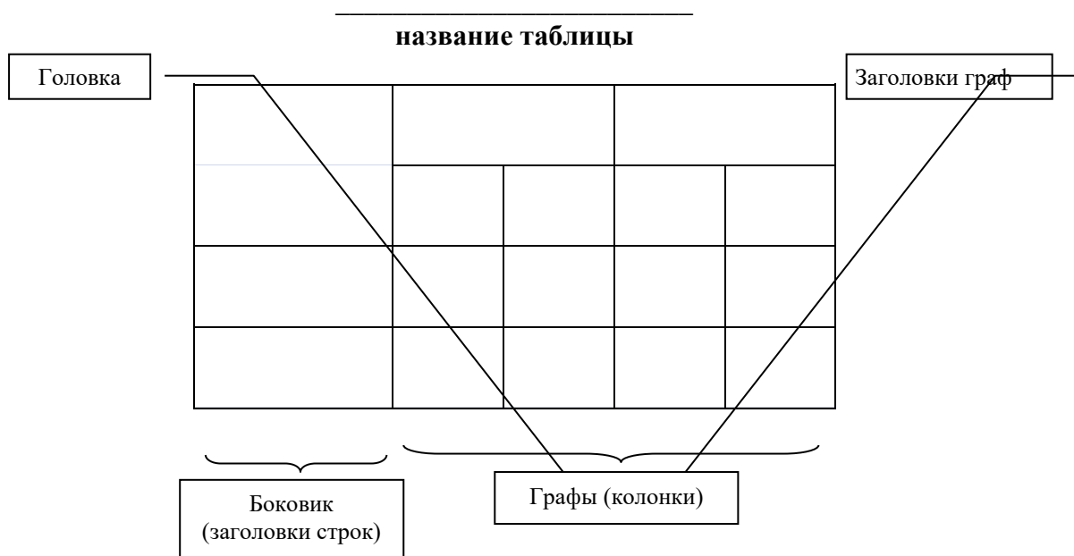
Рис. 1- Построение таблиц
